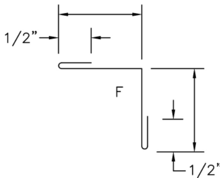
SOFFIT ANGLE
